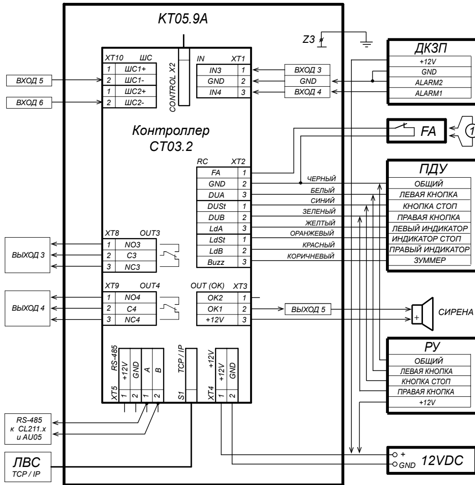
1 - переключатель-провод при отсутствии устройства Fire Alarm
